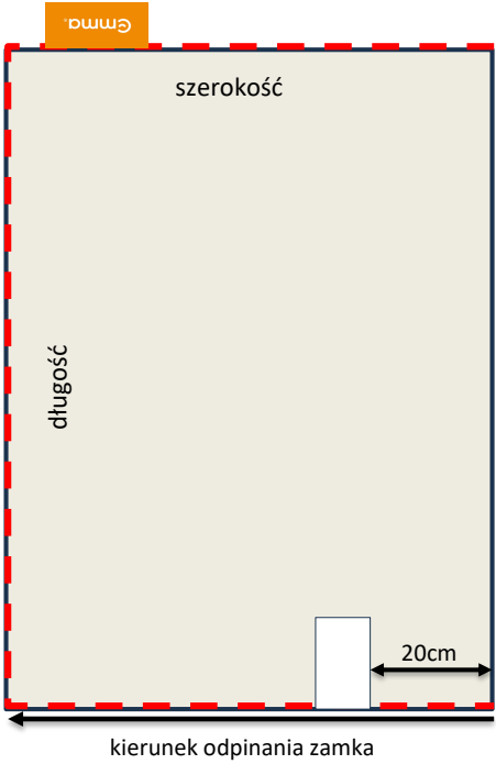
schemat szycia (zamek z 3 stron)
