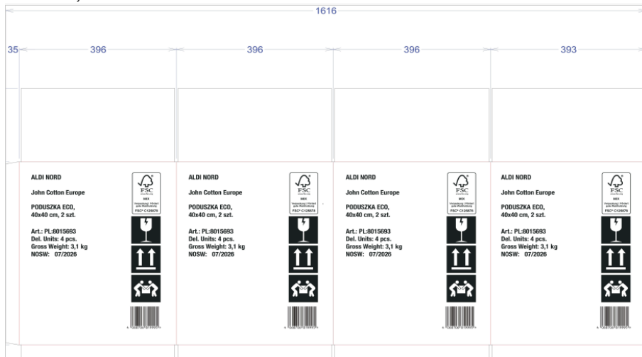
Karton zbiorczy
