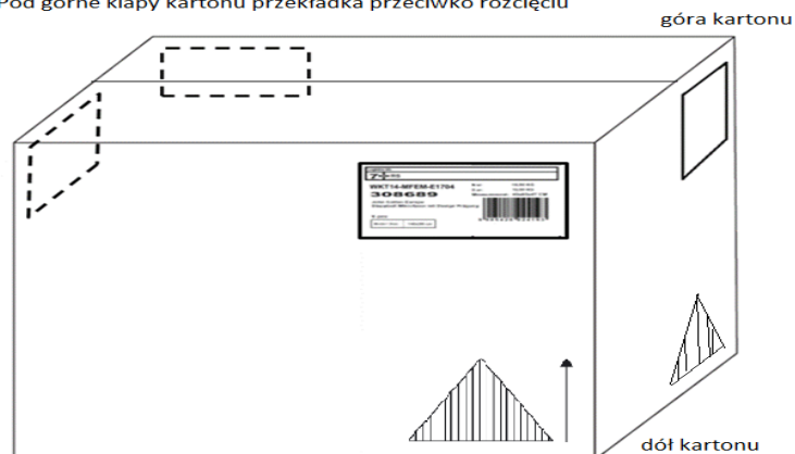
Podstawa trójkąta to dół kartonu
