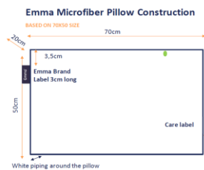
szcemat wszycia wszywki
