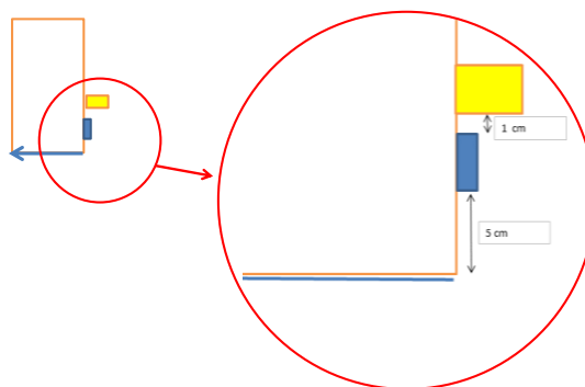
miejsce wszycia wszywek (strzałka oznacza pozycję suwaka po zamknięciu poszewki)
